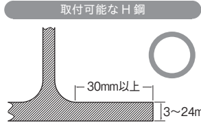
取付可能なH鋼
