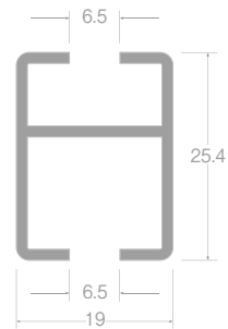
レール断面図 (単位: mm)
