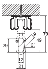
天井直付 (カラビナランナー使用)
