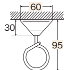
点滴フック寸法図（単位：mm）
