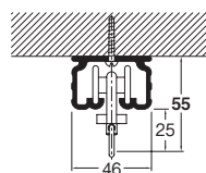
天井直付 (スイングランナー使用)
