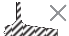
クリップ付ブラケットプレート取付面が傾斜になっている場合は、取付できません。
