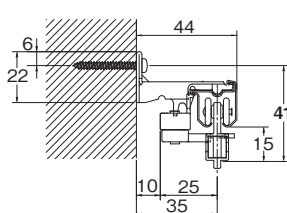
カバートップⅡセット平面図
