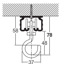
天井直付 (ヒートランナー使用)
