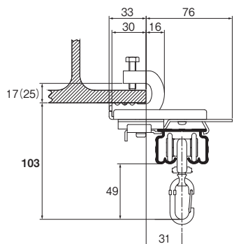
天井付シングルブラケットM 2 付 (持ち出し) (カラビナランナー使用)
